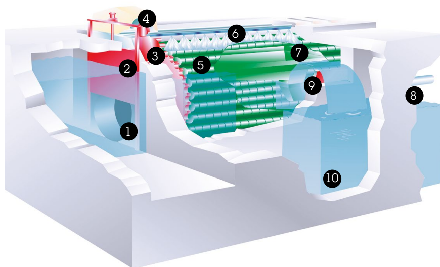
Funktionsablauf Trommelsieb RSH-M
